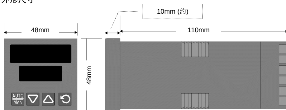
外形尺寸
